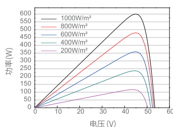
功率-电压曲线 JAM78D30-600/GB
