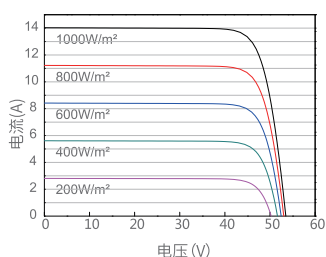
电流-电压曲线 JAM78D30-600/GB
