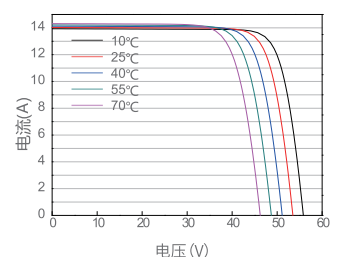
电流-电压曲线 JAM78D30-600/GB
